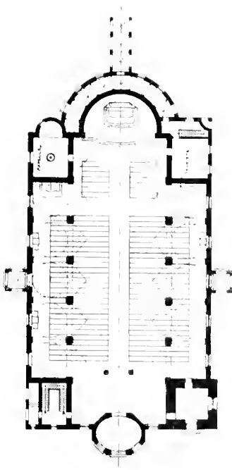
MOTTO «SKABIOSE» GRUNDRISS Nr. 26, Text S. N, vgl. Nr. 21, 25, 29
